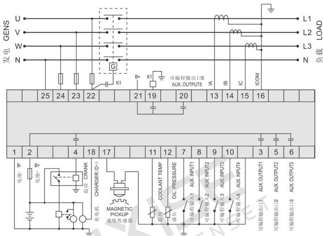
LXC3120 典型应用图
