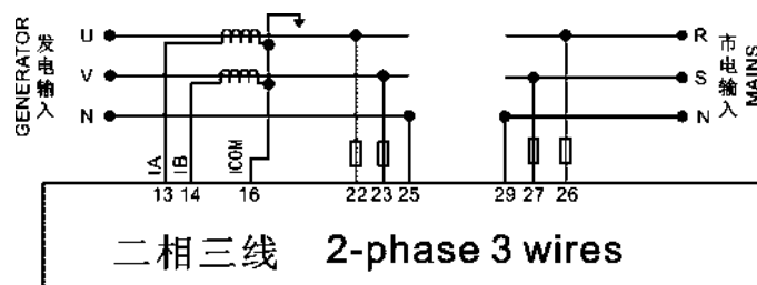
二相三线连接时接线图(以 LXC3120 为例)
